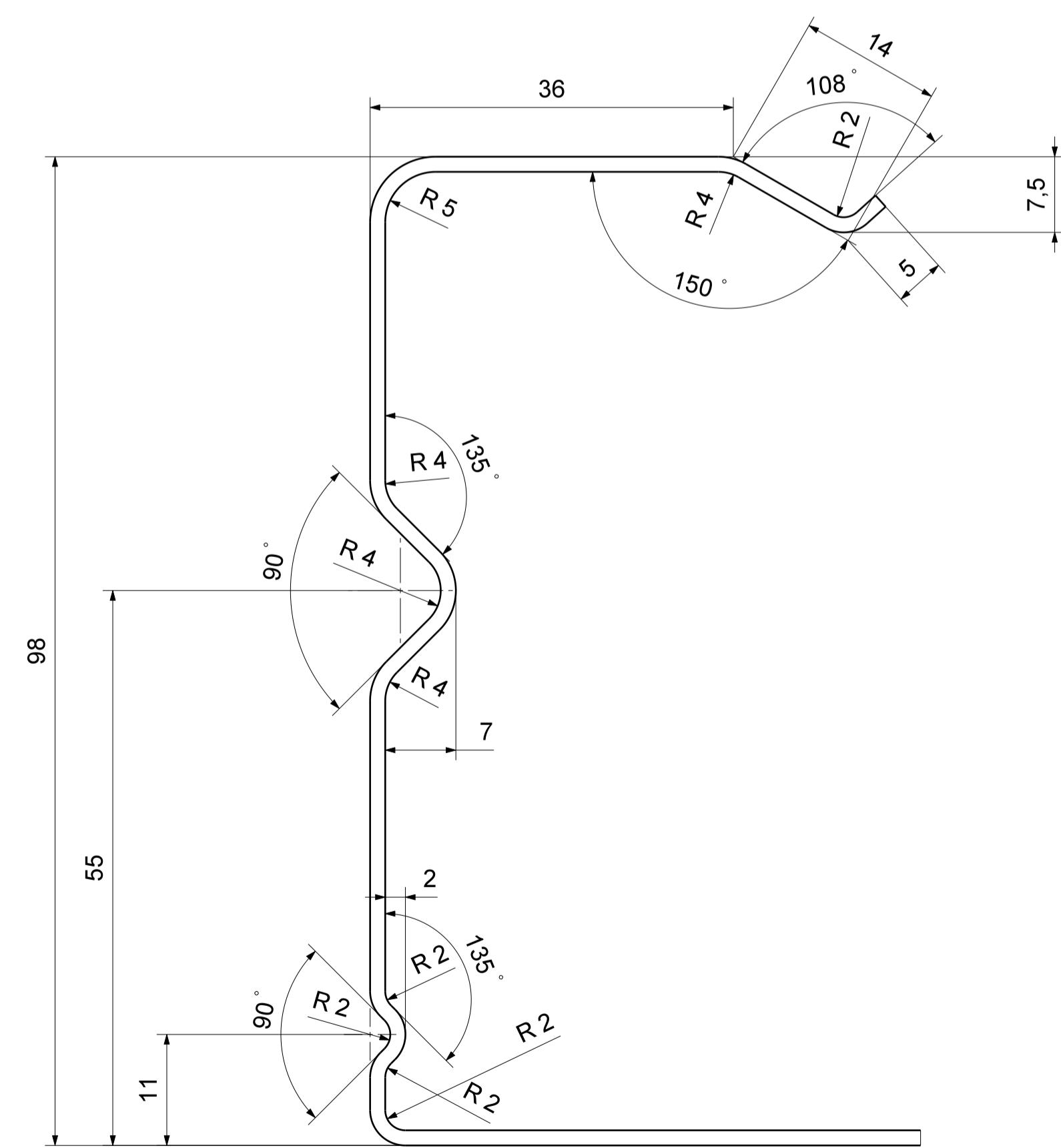
Detail B Maßstab: 2:1
