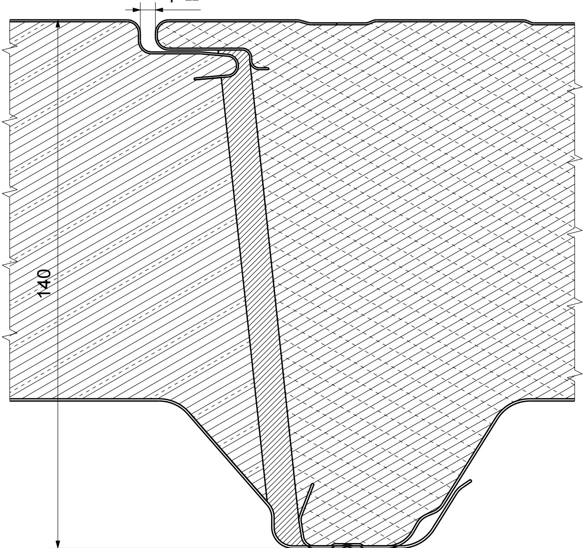
Vorderansicht Maßstab: 1:1
