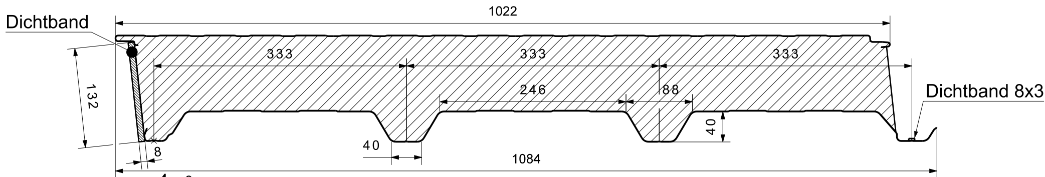
Vorderansicht Maßstab: 1:5
